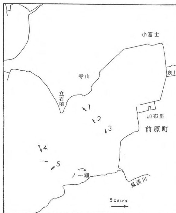
図5 恒流図
