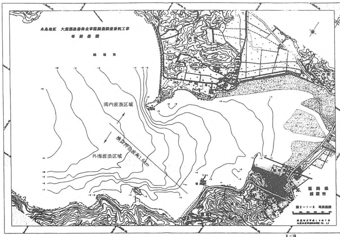
図3 等深线图
