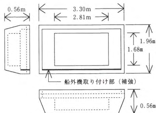
図2 摘採船の概要
