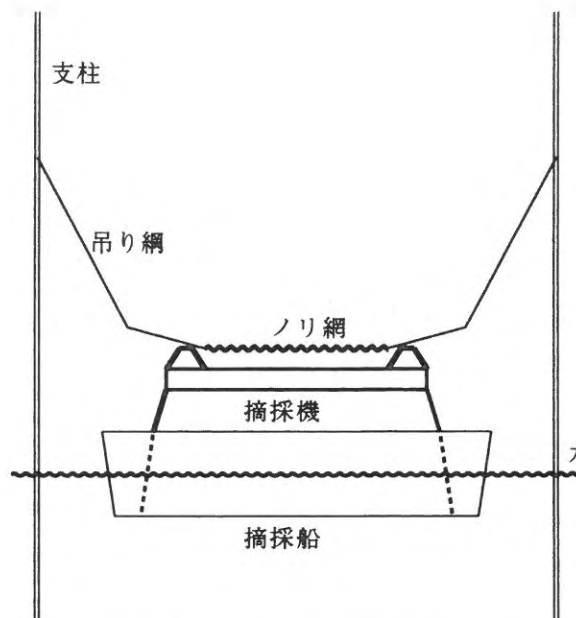
図6 摘採時のノリ網と吊り綱の関係
