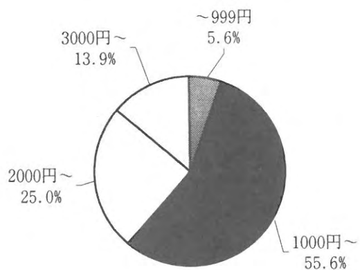
図7 ガザミ料理1品に払う金額
