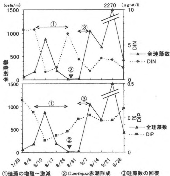
図3 栄養塩濃度とプランクトン発生状況の推移
