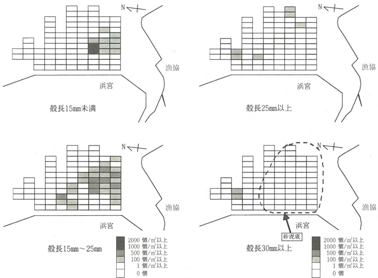
図3 椎田町浜宮地先における殻長別アサリ分布
