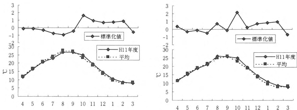
図3 水温の変化（左図：表層、右図：底層）
