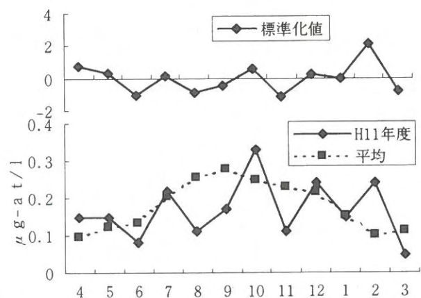
図7 PO 4 -Pの変化 (左図：表層、右図：底層)
