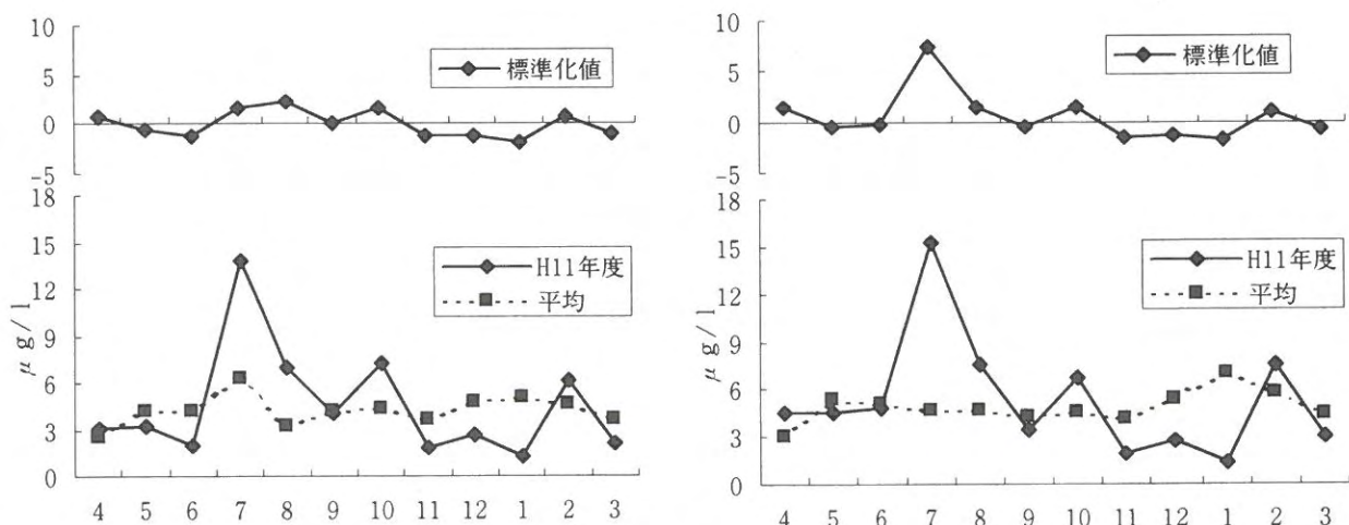
図10 Chl-aの変化 (左図：表層、右図：底層)
