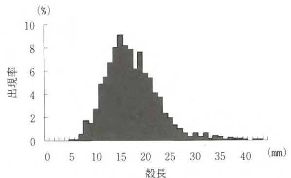
図2 アサリ殻長組成
