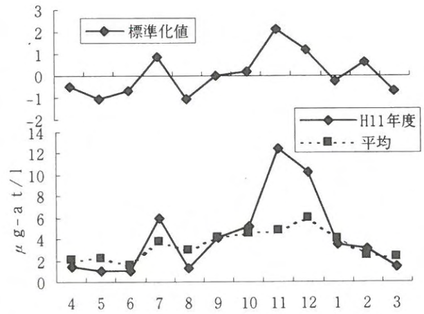
図6 DINの変化 (左図：表層、右図：底層)
