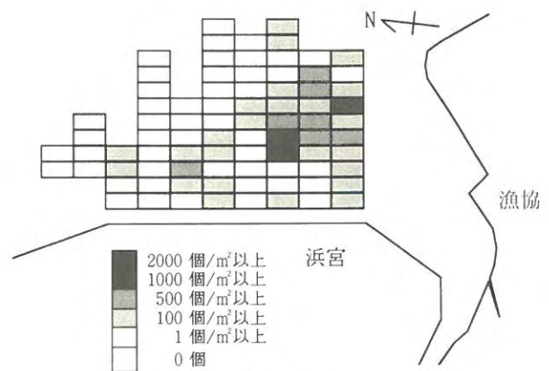
図1 椎田町浜宮地先におけるアサリの分布
