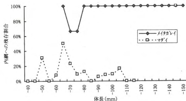
図16 選別網における内網への残存割合
