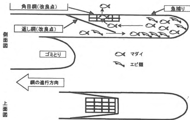
図17 幼魚混獲防止網模式図（網後部）
