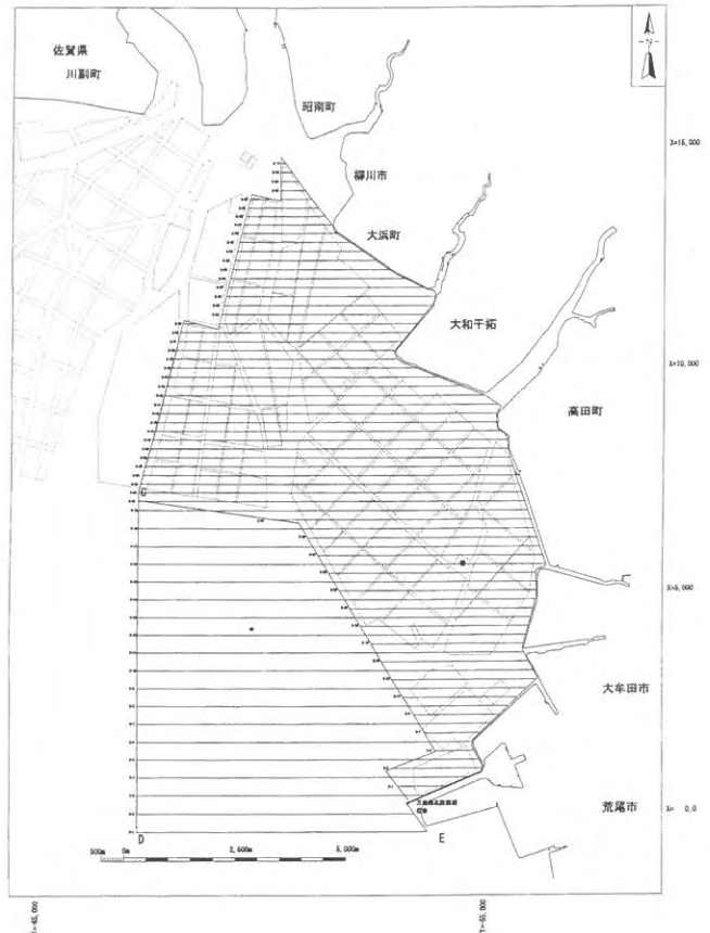
図1 測量区域図
