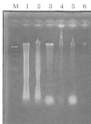
図2 異なる前処理と抽出法の組み合わせによるノリ葉体からのDNA抽出 左：キアゲンチップ処理前 右：キアゲンチップ処理後
