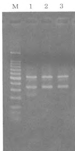
図7 同一品種の板ノリと葉体から抽出したDNAのRAPDの比較 1・2:板ノリから抽出したDNA 3:葉体から抽出したDNA M:100bpマーカー
