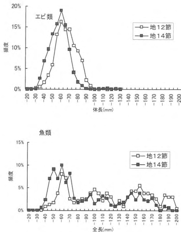
図5 体長別頻度
