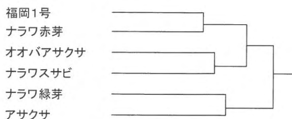
図10 BSIから求めた養殖品種間の類似度関係図
