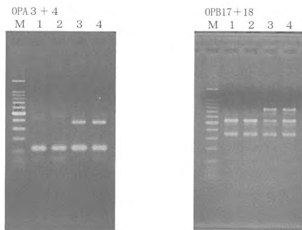
図5 2分したノリ葉体2個体から抽出したDNAのRAPD泳動像 1・2:個体A 3・4:個体B M:100bpマーカー
