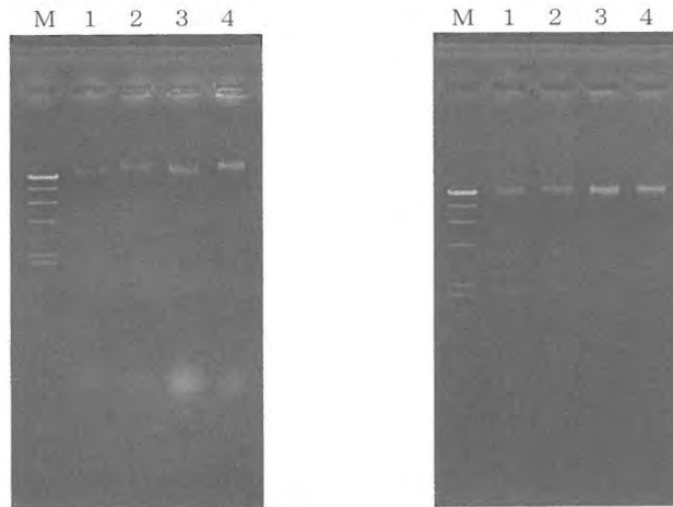
図3 ISOPLANTとISOPLANT IIのDNA抽出効率の比較 左:キアゲンチップ処理前 右:キアゲンチップ処理後 1・2:ISOPLANT 3・4:ISOPLANT II M:マーカー( \lambda -HindIII)
