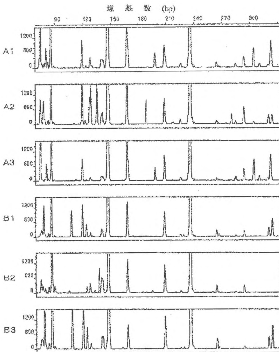
図9 同じサンプルを使ったAFLPフィンガープリントパターン
