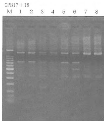
図6 ノリ葉体から抽出したDNAのRAPD再現性 1~6:加布里養殖葉体 7・8:姪浜養殖葉体 M:100bpマーカー
