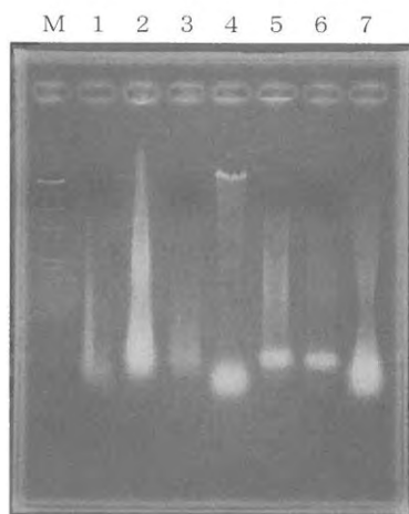
図1 異なる前処理と抽出法の組み合わせによるノリ葉体からのDNA抽出
