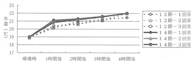
図15 発泡容器中の海水の水温変化
