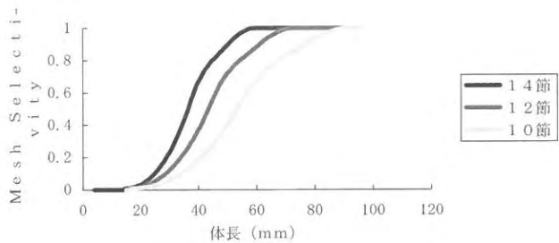
図27 サルエビの網目選択性曲線
