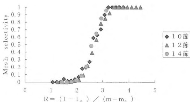
図23 Rに対する網目選択率 (アカエビ)
