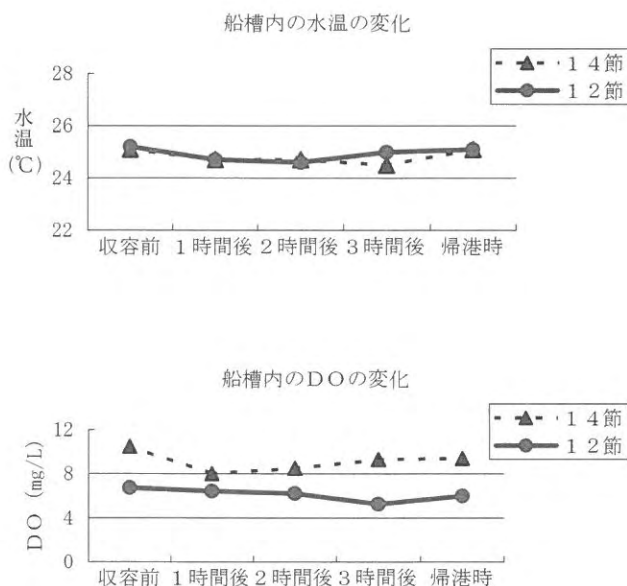
図11 操業中の船槽内の水温、DOの変化
