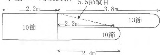
図3 けた網試験漁具の概要図
