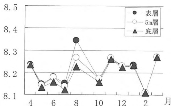
図6 pH の変化
