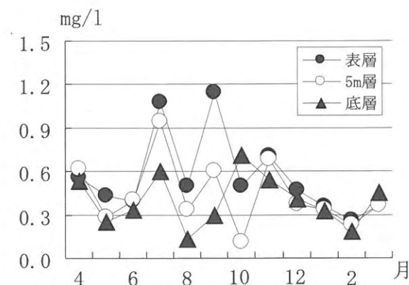
図5 COD の変化
