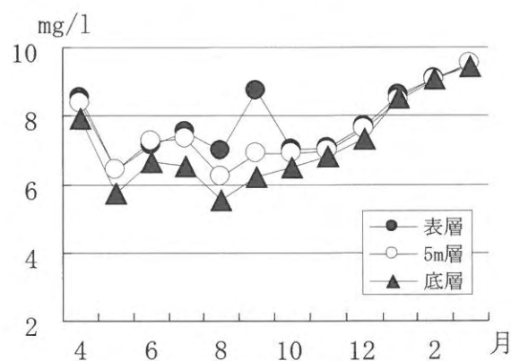
図4 DO の変化
