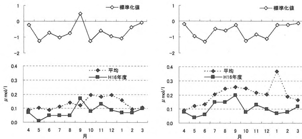
図6 \text{PO}_4\text{-P} の変化
