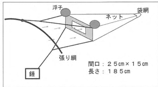
図2 稚魚ネット概略図
