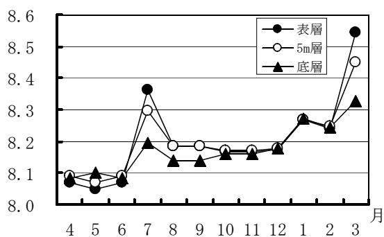
図6 pHの変化
