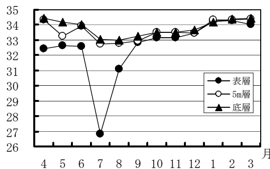
図3 塩分の変化
