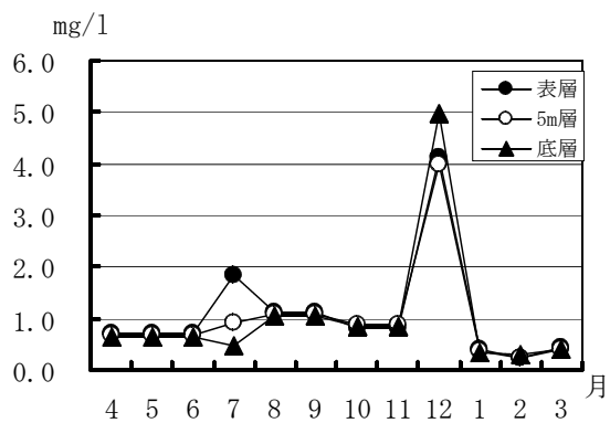
図5 CODの変化
