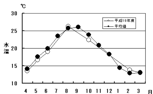
図3 水温の変化
