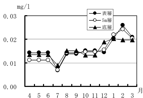
図8 TNの変化
