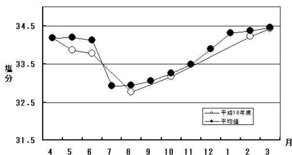
図4 塩分の変化
