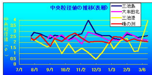
図 12 定点追跡調査 表層中央粒径値の推移
