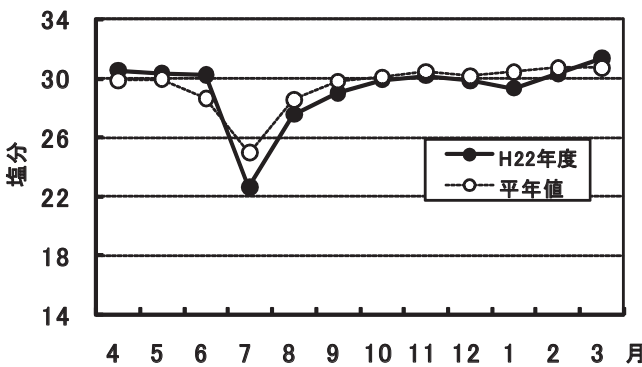
図3 塩分の推移
