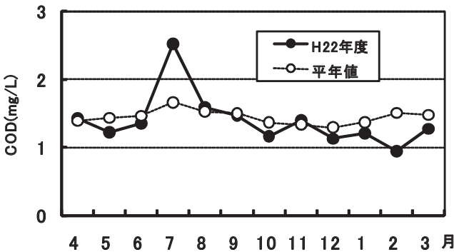
図5 CODの推移
