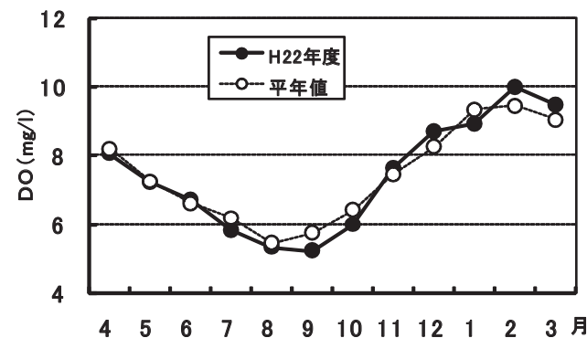
図4 DOの推移
