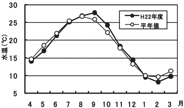
図2 水温の推移
