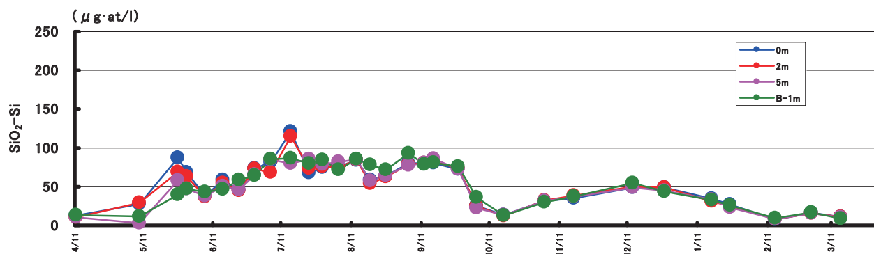
図10 \text{SiO}_2\text{-Si} の推移 (B3)
