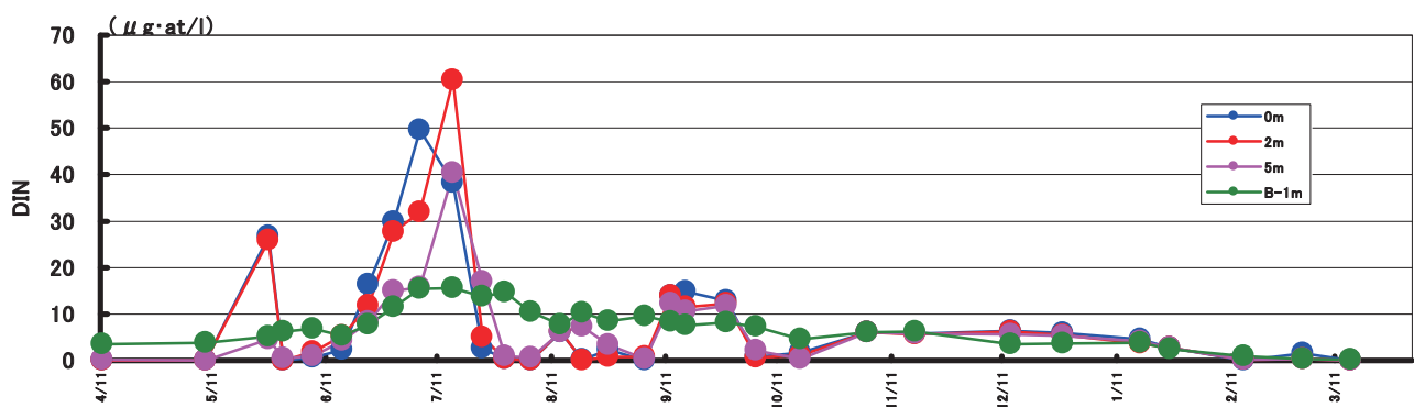
図3 DINの推移 (P1)
