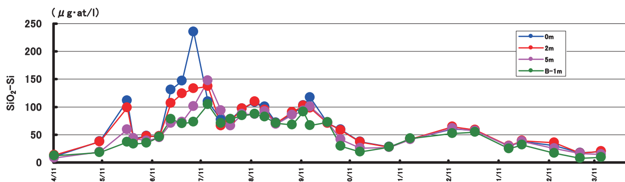
図12 \text{SiO}_2\text{-Si} の推移 (P6)
