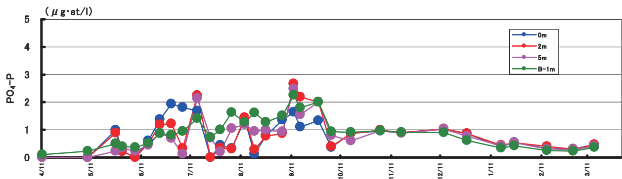
図8 \text{PO}_4\text{-P} の推移 (P6)
