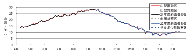
図 18 1 日平均水温の推移
