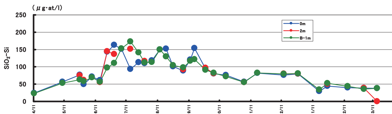
図13 \text{SiO}_2\text{-Si} の推移 (T2)
