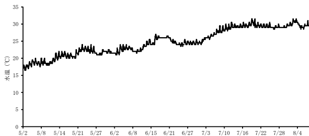
図7 水温の推移
