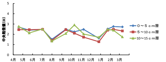
図 36 竹ハゼ南漁場における中央粒径値の推移
