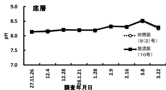
図5 pHの推移
