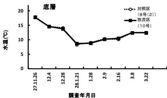
図3 水温の推移
