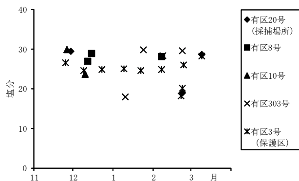
図34 塩分の推移
