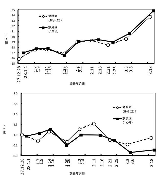
図10 乾ノリの色
