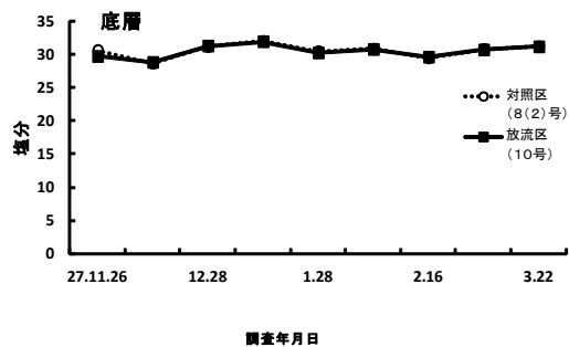
図4 塩分の推移
