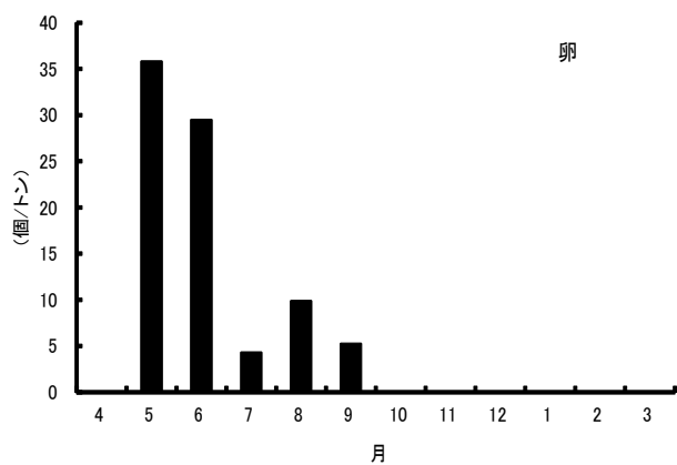
図2 カタクチイワシ卵及び稚仔の月別出現状況（1調査点当たりの平均値）
