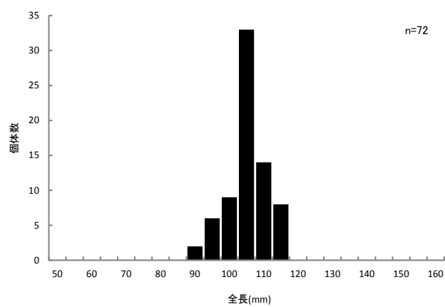
図 5 シャコの全長組成
