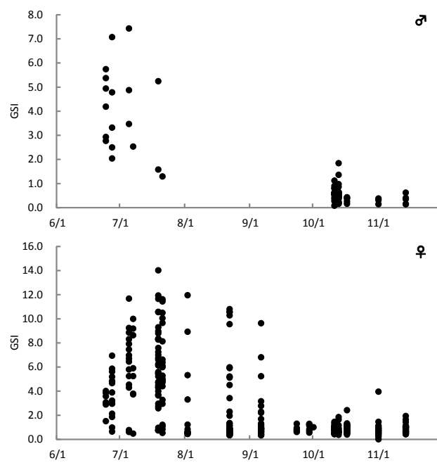
図 6 GSIの推移
