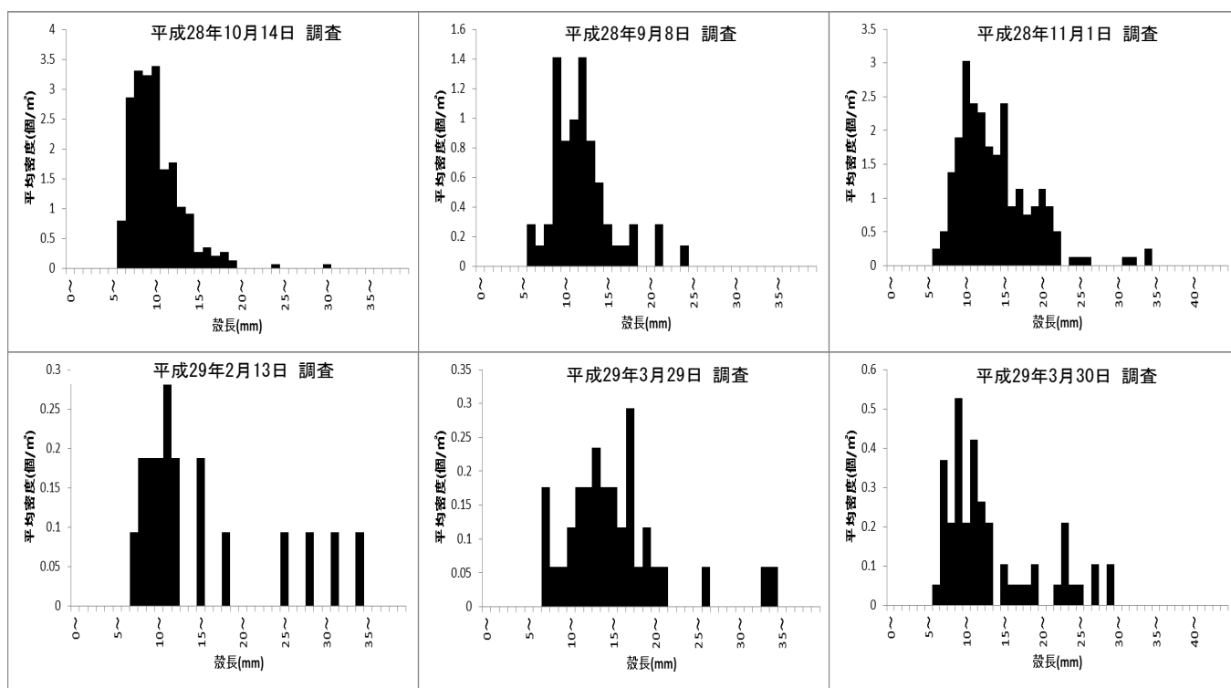
図5 アサリ殻長組成（蓑島）
