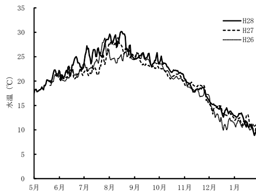
図 6 水温の推移
