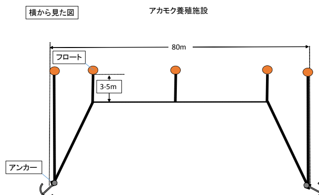
図2 アカモク養殖試験施設
