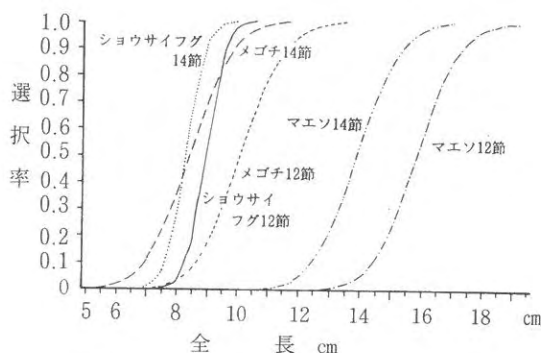
図24 小型底びき網の魚種別選別率
