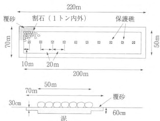
図1 マナコ増殖場の構造
