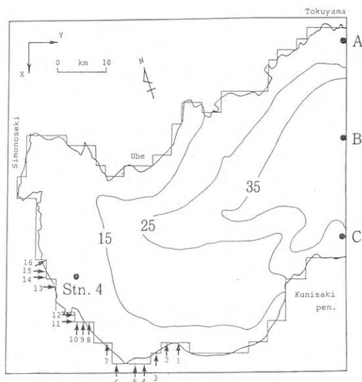
図9 計算領域
