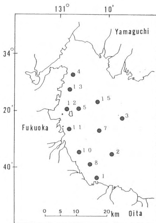
図1 海洋調査点
