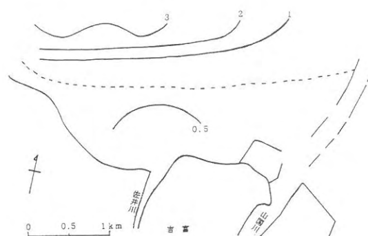
図4 強熱減量 (%)
