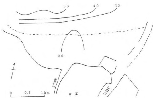
図3 水分 (%)
