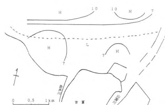
図7 C/N比
