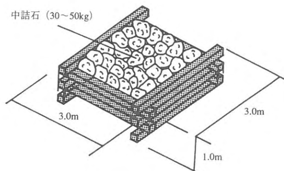
図20 稚貝保護礁の形状
