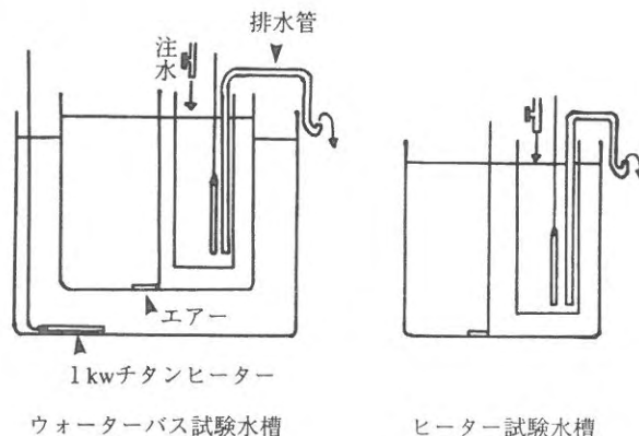
図1 仔魚飼育槽の模式図
