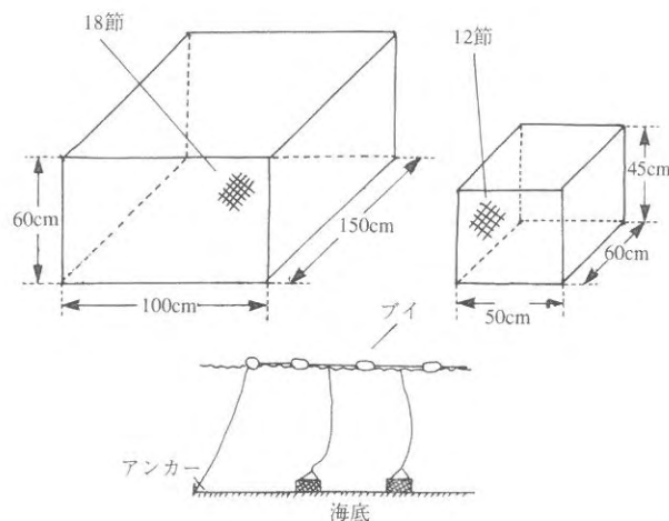
図6 ナマコ養殖施設模式図
