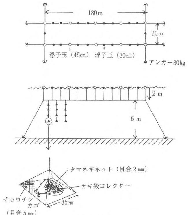
図2 中間育成施設図
