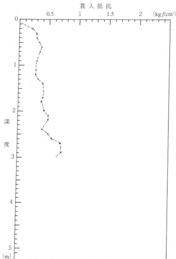
図3 深度別コーン貫入抵抗 q_c ( \text{kgf/cm}^2 )
