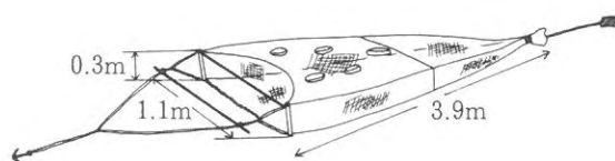
図8-1 潜底式試験定置網 (St. 1)
