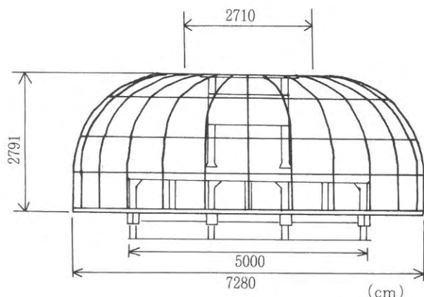
図2 改良型魚礁構造図（シーボリスB3型）
