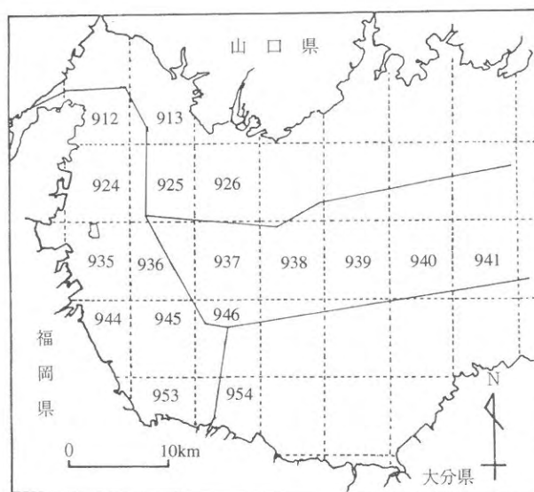
図15 海区番号図
