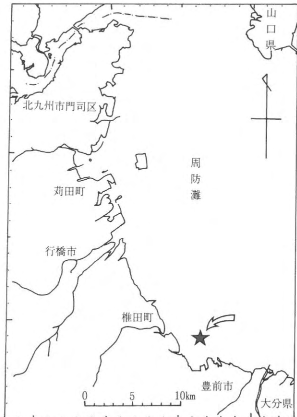
図1 調査海域図
