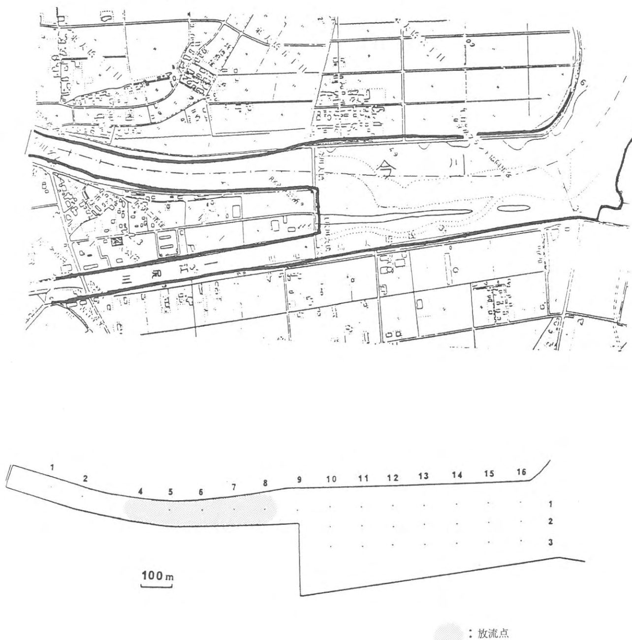
図2 調査定點
