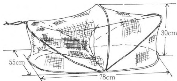
図8-3 えびかご (St. 3～8)
