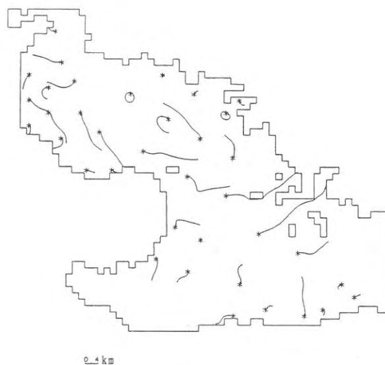
図1-5 計算された流れにトレーサを投入し、1週間漂流させた結果 (*印は始点を表す)
