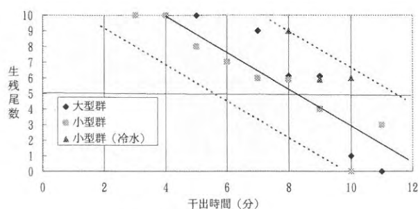
図3 マダイ幼魚の干出耐性試験
