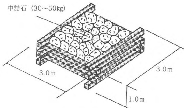
図 6 稚貝保護礁の形状
